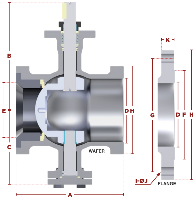
Dimensions - ASME 150 / 300
